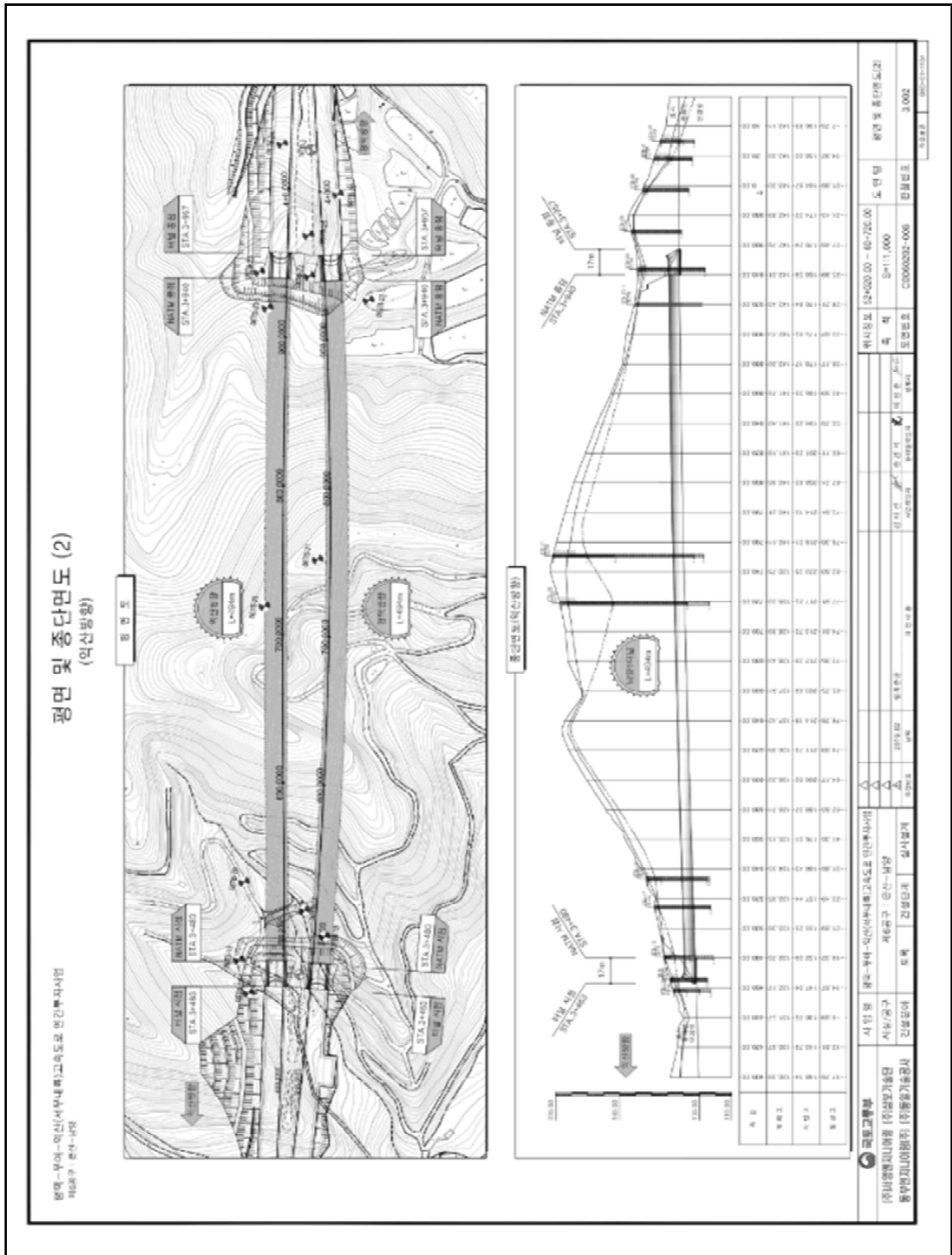
【그림 2.17.2】 평면 및 종단면도
